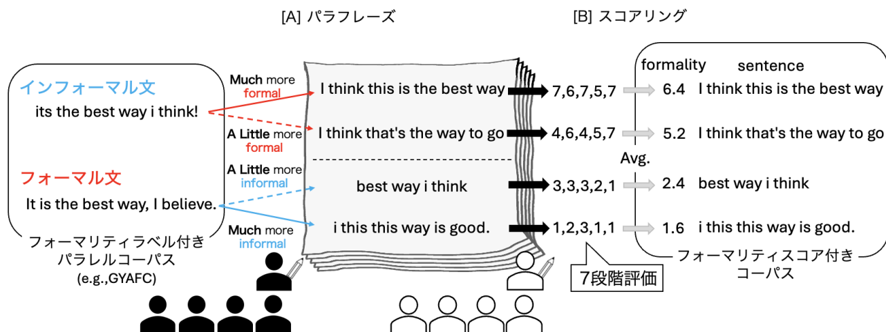
図1 提案手法：フォーマリティスコア付きコーパスの収集
